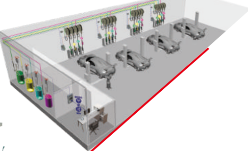
Brake bleeder 刹车油更换机
